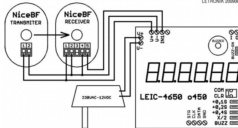
Schemat systemu z czujnikiem Nice BF
